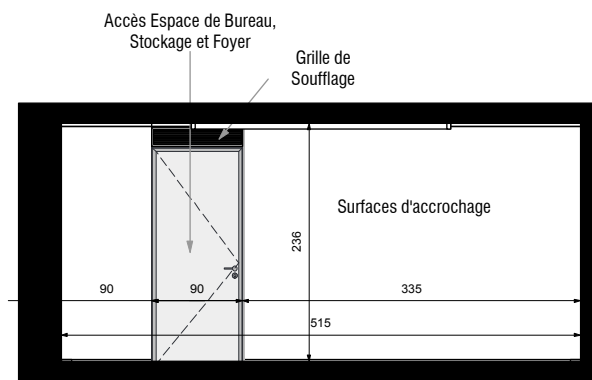
COUPE EE
